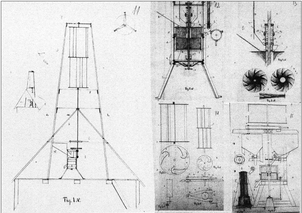
15 pav. A. Diržio automatinis vėjo malūnėlis
