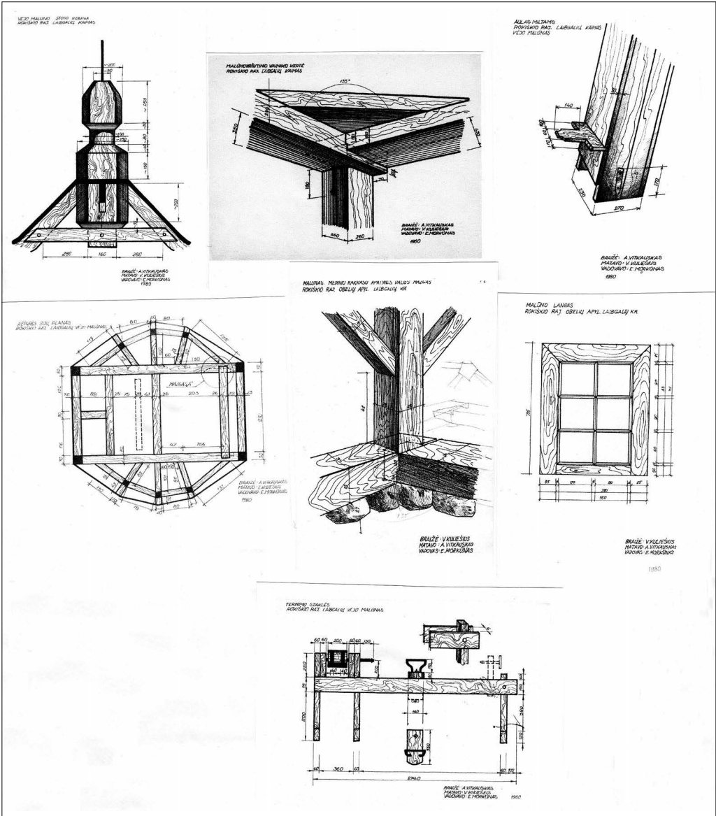
4 pav. Kaulino motorinio malūno mazgai
