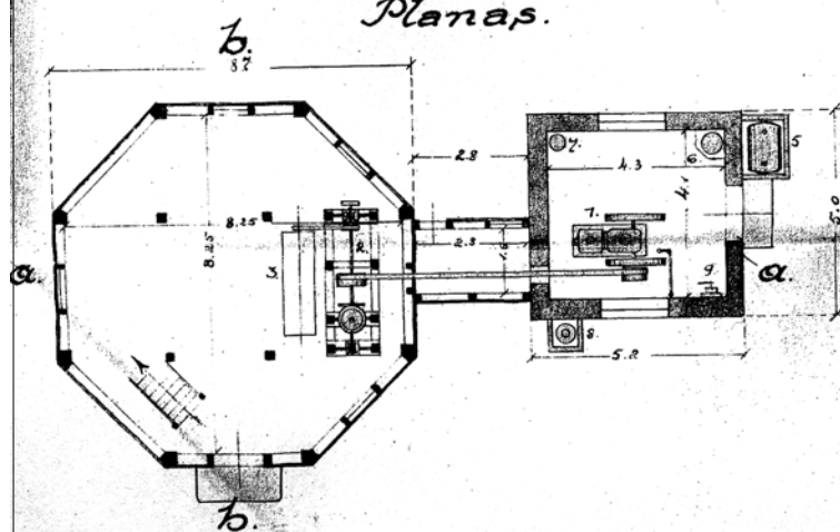
Planas.
